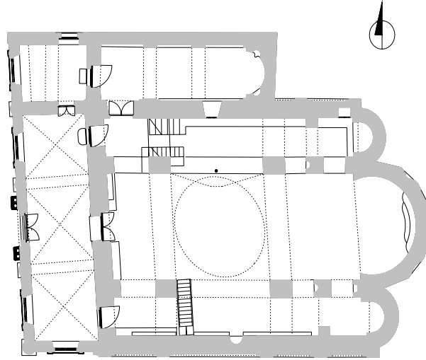
Şekil 2. Hagios Gregorios Theologos Kilisesi zemin kat planı
