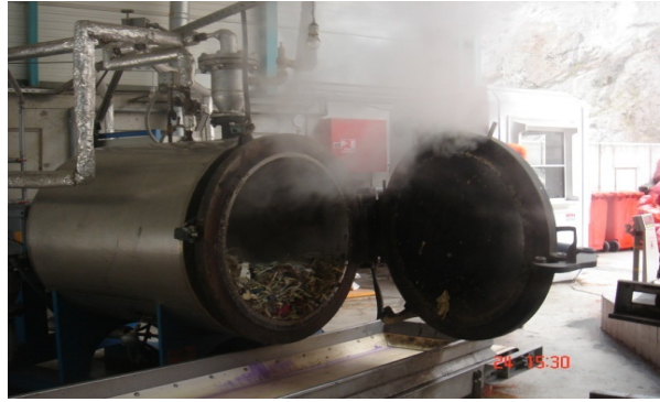
Şekil 5. Trabzon/Dikilitaş mevki Transfer istasyonundaki Sterilizasyon Ünitesi[]
