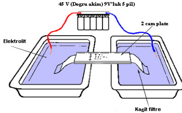
Şekil 2. Düşük gerilimle çalışan kâğıt elektroforez düzeneği. Kâğıt tampon çözelti ile doyurulduktan sonra, iki ucu tampon çözeltiye batacak şekilde gerilir. Örnek madde kâğıt üzerine genellikle bir çizgi halinde sürülür. Kurumaması için kâğıt hem üstten kapatılır hem de bir su deposu üstünde tutulur. Gerilim uygulandıktan sonra bir süre bekletilir, süre tamamlandığında kâğıt çıkartılır, kurutulur ve analiz edilir.
