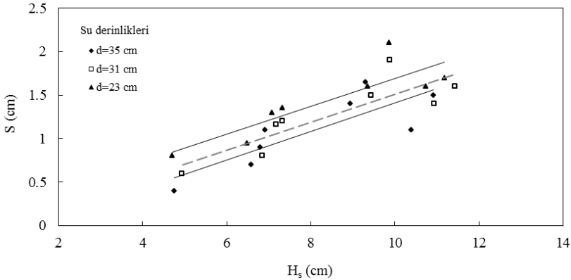
Şekil 7. Oyulma derinliğinin belirgin dalga yüksekliği ve su derinliği ile değişimi
