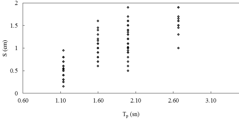
Şekil 6. Oyulma derinliğinin pik dalga periyodu ile değişimi
