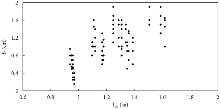
Şekil 5. Oyuлма derinliğinin ortalama dalga periyodu ile değışimi
