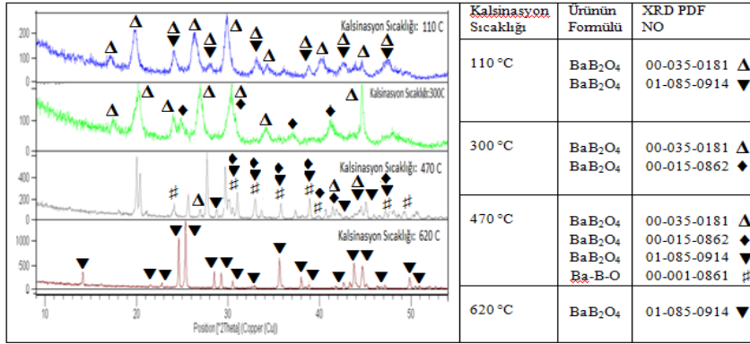
Şekil 3.6. Farklı sıcaklıklarda kalsine edilen numunelerin XRD analiz sonuçları
