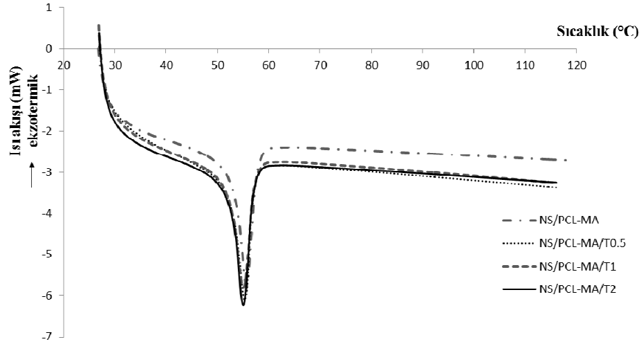
Şekil 4. NS/PCL-MA ve kompozit örneklerinin DSC diagramlarında 2. ısıtma eğrileri
