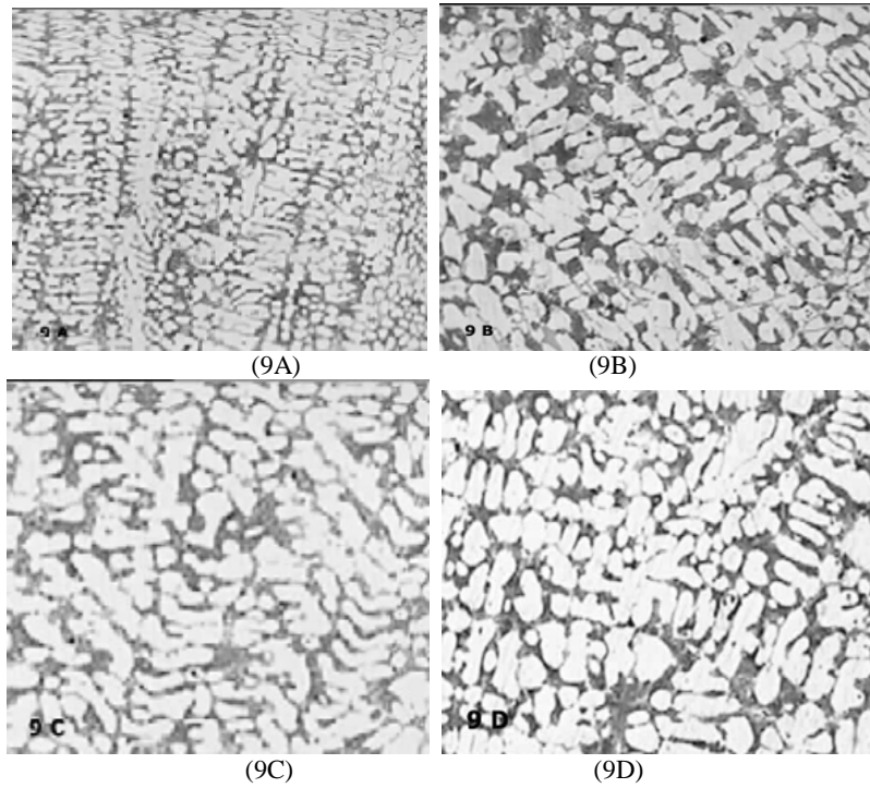
Şekil 5. 9 numaralı döküm parçasından alınmış mikroyapı görüntüleri
