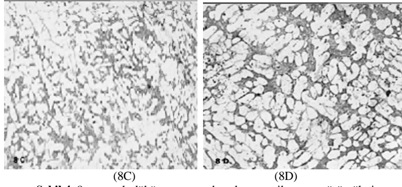
Şekil 4. 8 numaralı döküm parçasından alınmış mikroyapı görüntüleri
