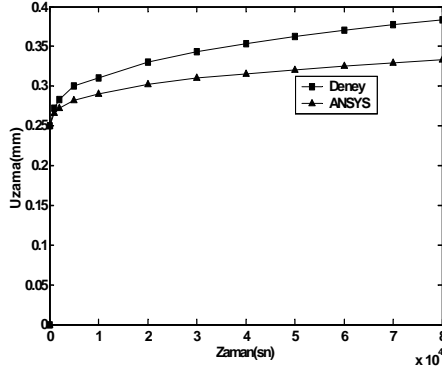
Şekil 11-a) 1,757 MPa gerilme altında deney ve dört gerilme durumu için ANSYS değerleri
