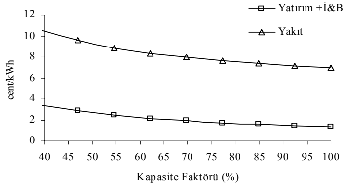
Şekil 8. T_3= 1100 K ve P_{rc}=14 olduğu durumda kapasite faktörü ile masraf gruplarının değişimi
