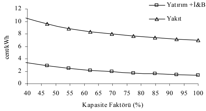
Şekil 8. T_3=1100\text{ K} ve P_{rc}=14 olduğu durumda kapasite faktörü ile masraf gruplarının değişimi
