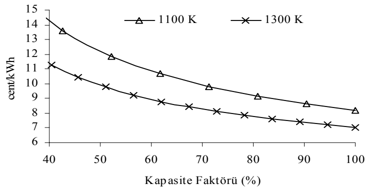
Şekil 10. P_{rc}=14 olduğu durumda kapasite faktörü ile birim elektrik maliyeti değişimi
