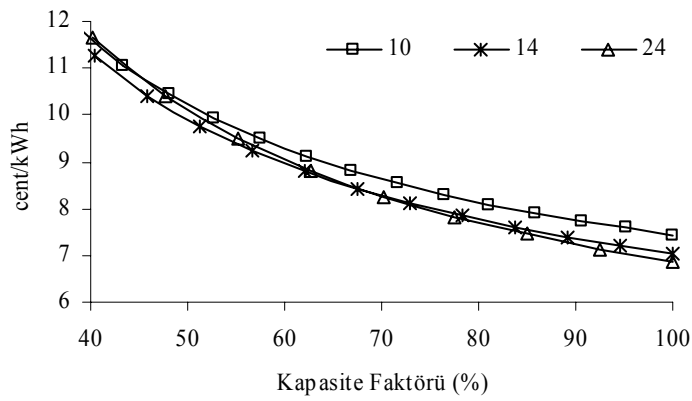
Şekil 9. T_3= 1300 K olduğu durumda kapasite faktörü ile birim elektrik maliyeti değişimi
