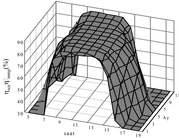
Şekil 8. Seçilen sistem veriminin hesaplamalarda kullanılan panelin maksimum çalışma noktalarındaki (MPP) verimine oranının saat ve aylara göre deđişimi
