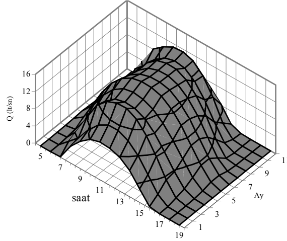
Şekil 7. Pompalanan su debisinin saat ve aylara göre deđişimi
