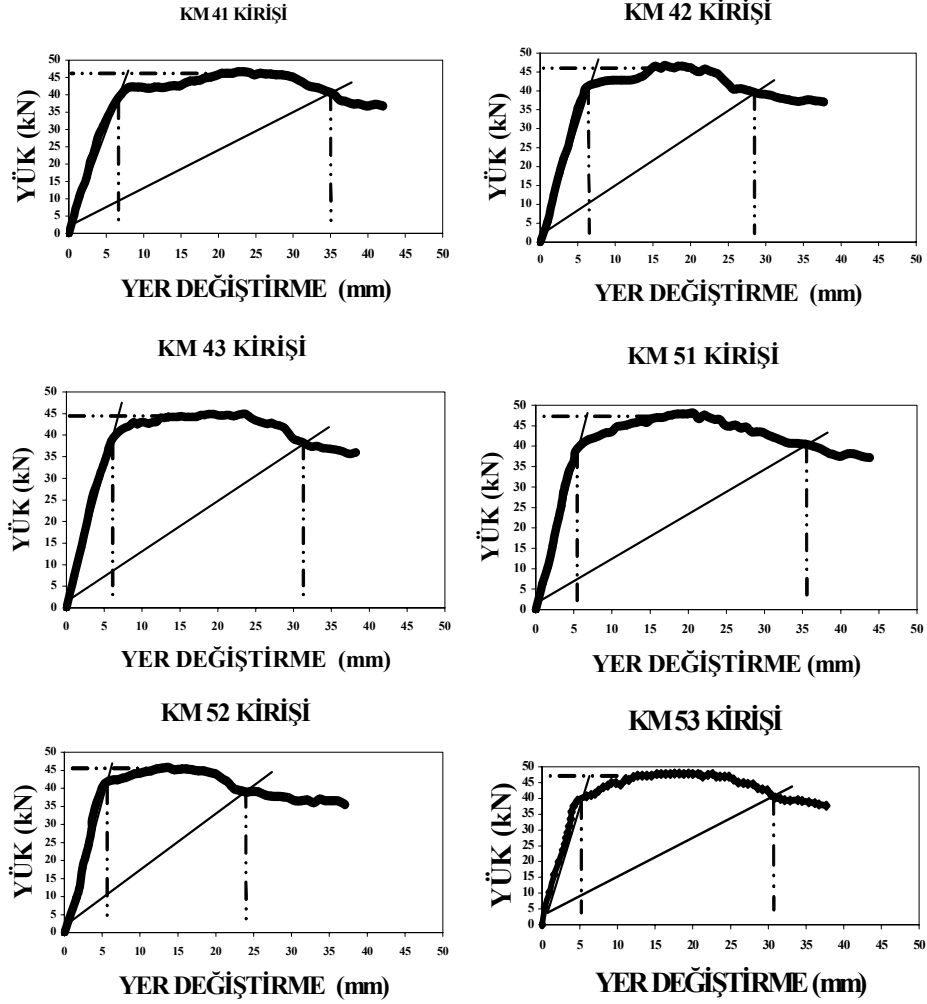
Şekil 5. Betonarme mantolama ile güçlendirme yapılmış kirişlerin yük- yer değiştirme eğrileri (KM4 ve KM5 serisi kirişler)
