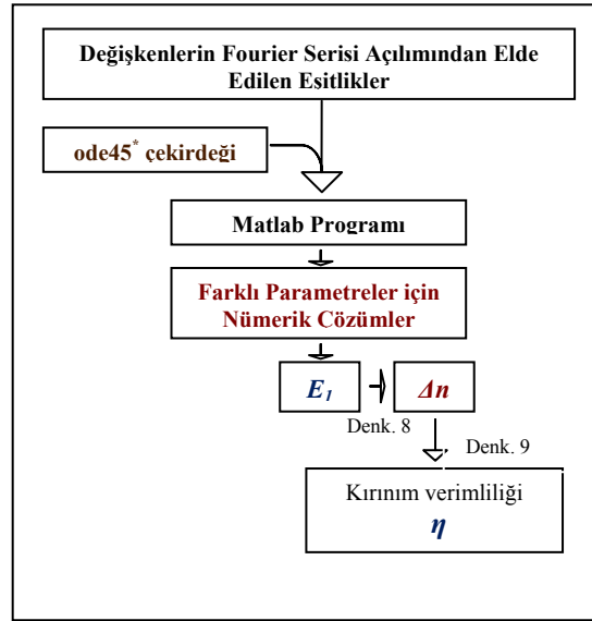
Şekil 2. Yapılan hesaplamaların akış diyagramı
