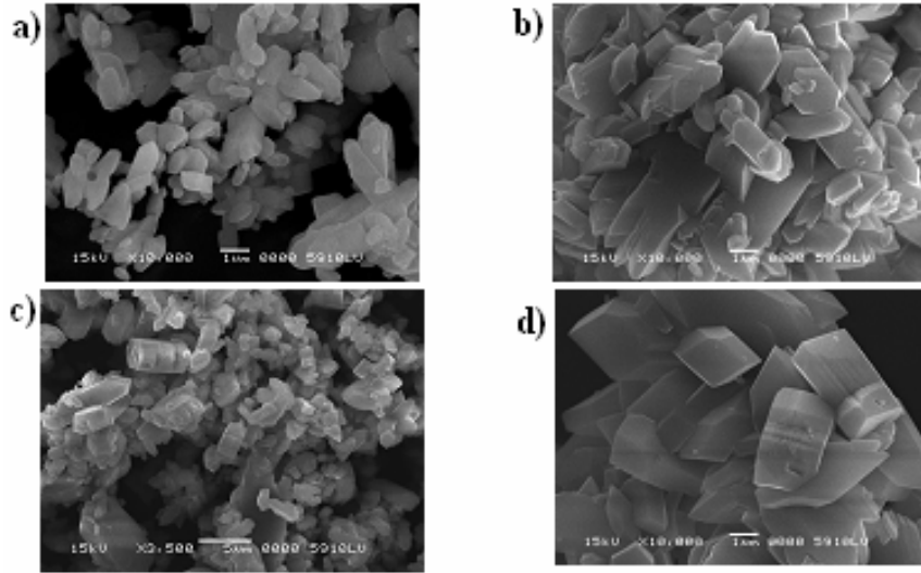
Şekil 7. Kristallere ait SEM Fotoğrafları Diyagramları a) COM aşı kristalleri, b) Katkı maddesi olmadan elde edilen kristaller, c) Polimer B varlığında elde edilen kristaller, d) PAA homopolimeri varlığında elde edilen kristaller
