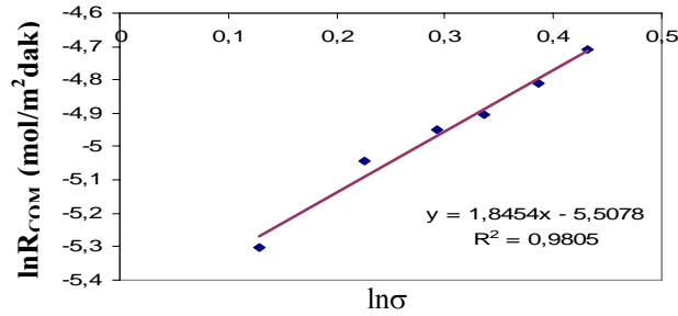
Şekil 3. Relatif aşırı doyumluğun COM kristalizasyon hızına etkisi ( T_{Ca}/T_{OX}=1 , T_{NaCl}=0.1 mol/l, 0.1g/L polimer B, T=37 °C)
